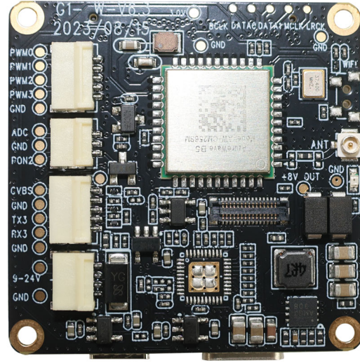
Rückansicht
